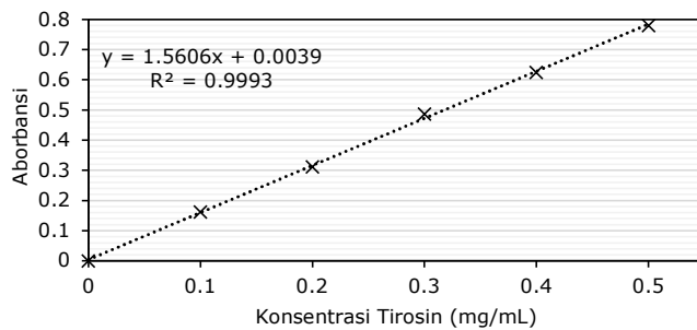
Gambar 1. Kurva Standar Tirosin
