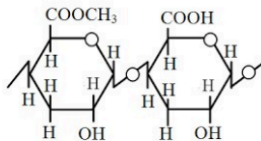
Gambar 3. Struktur Senyawa Pektin
