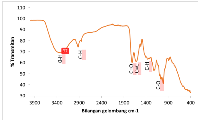
Gambar 2. Spektrum IR Ekstraksi Pektin
