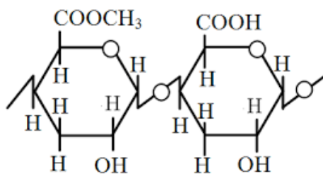
Gambar 3. Struktur Senyawa Pektin
