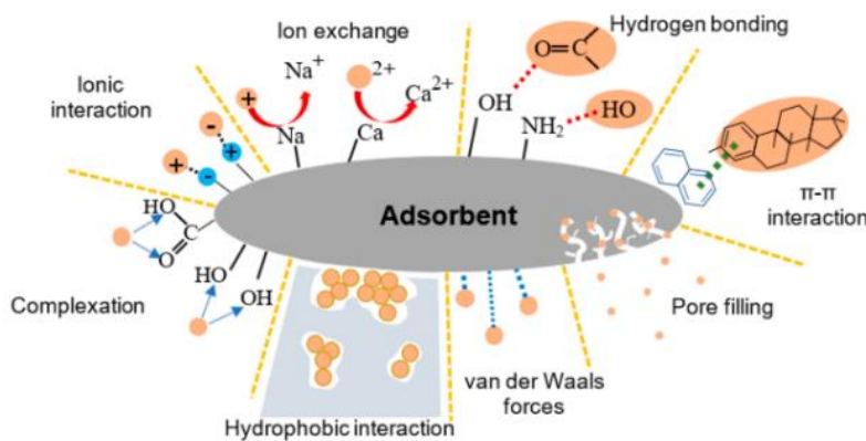
Gambar 4. Mekanisme Adsorpsi oleh Material Berpori Berbasis Pektin
