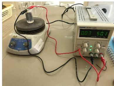
Gambar 4. Proses Anodisasi Ti
