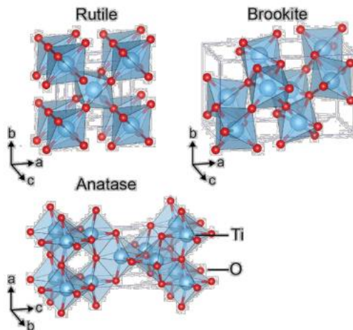
Gambar 1. Bentuk kristal TiO 2 (Setyawan & Suryani, 2024).
