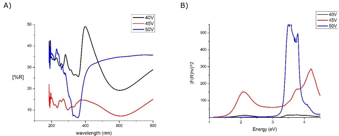
Gambar 6. A) Spektrum UV-Vis DRS TNAs Variasi Potensial. B) Tauc Plot TNAs Variasi Potensial
