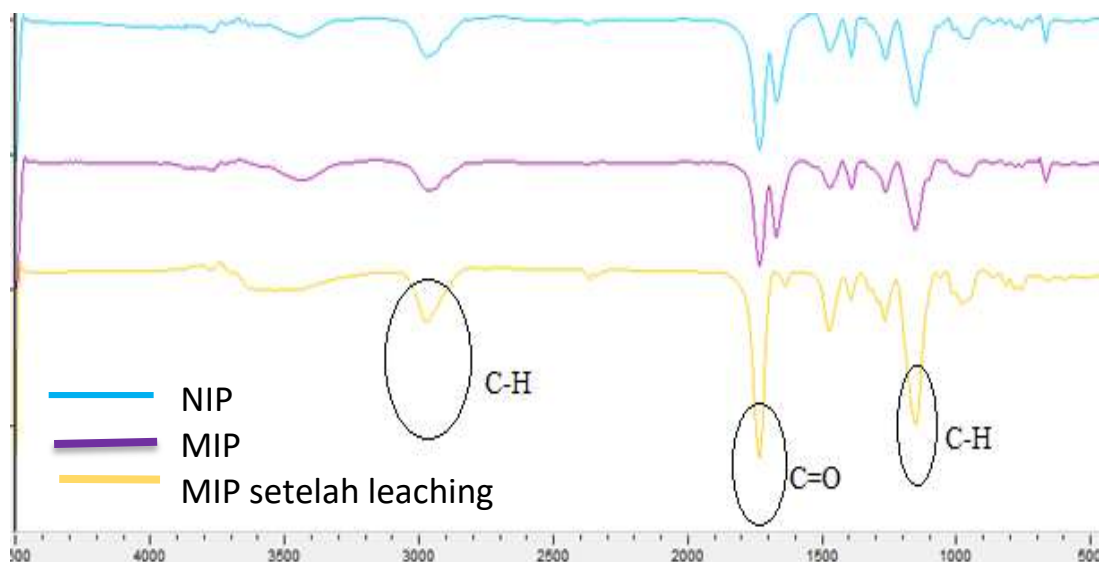
Gambar 3.3. hasil FTIR MIP, NIP dan MIP Leaching
