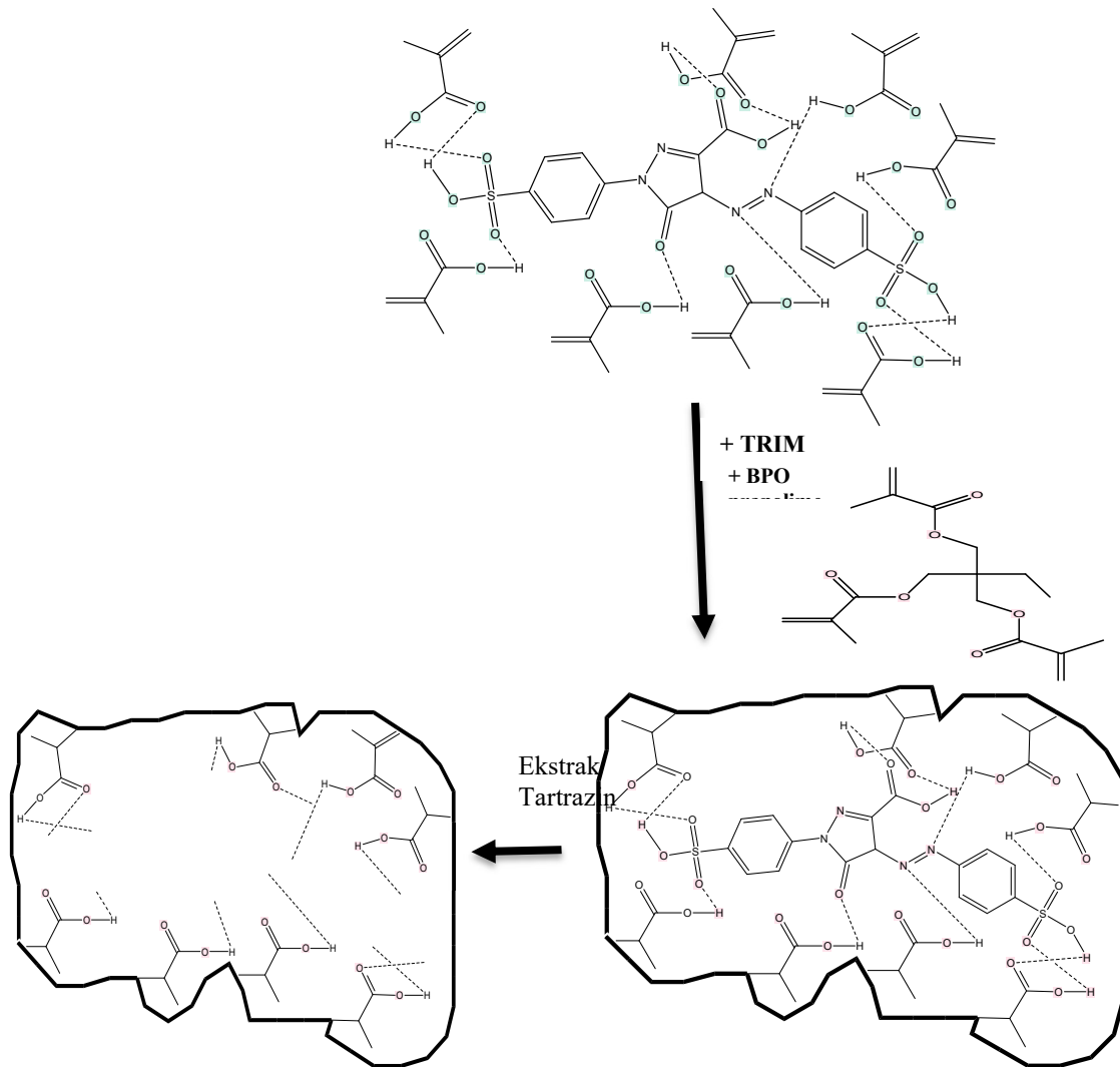
Gambar 3.3 Skema Sintesis Polimer Bercetakan Molekul Tartrazin
