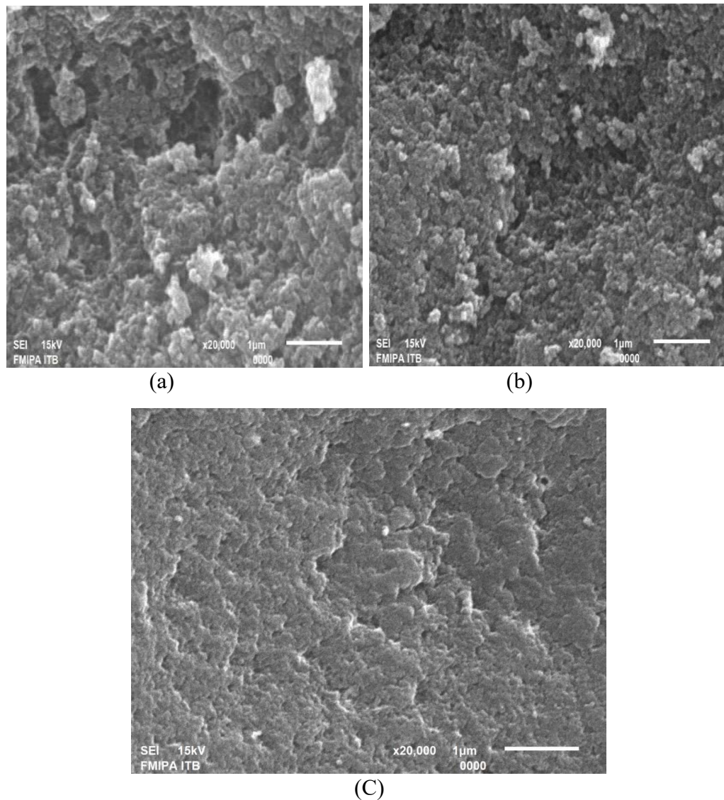
Gambar 3.5 Morfologi permukaan NIP (a) , Tartrazin-IP (b), Tartrazin-IP setelah ekstraksi molekul cetakan dengan methanol :ammonia (9:1) dengan perbesaran 20.000x (c)
