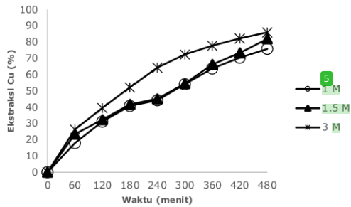
Gambar 5. Profil persen ekstraksi tembaga sebagai fungsi waktu pada berbagai konsentrasi peroksida
