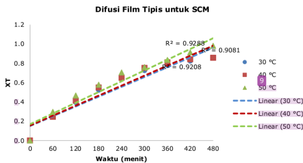
Gambar 8. Grafik X_T vs t pada berbagai temperature
