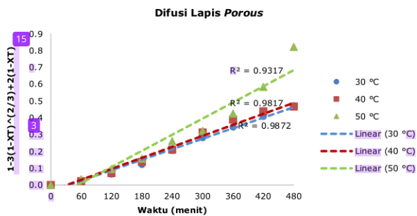
Gambar 9. Grafik (1-3(1-X_t)^{2/3}+2(1-X_t)) vs t pada berbagai temperature
