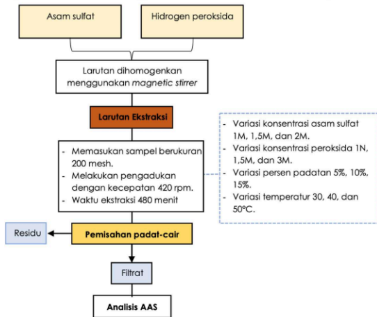
Gambar 1. Diagram alir proses ekstraksi
