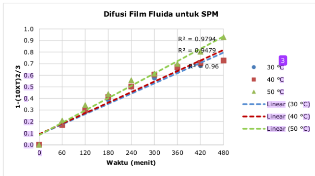
Gambar 11. Grafik 1-(1-X_T)^{2/3} vs t pada berbagai temperatur
