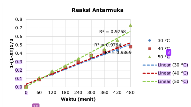
Gambar 10. Grafik 1-(1-X_t)^{1/3} vs t pada berbagai temperature
