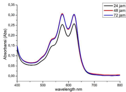
Gambar 5. Spektrum UV-Vis ekstrak bunga telang
