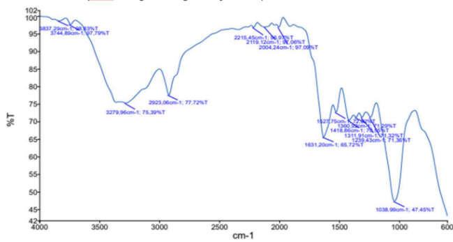
Gambar 4. Identifikasi gugus fungsi bunga telang dengan FTIR
