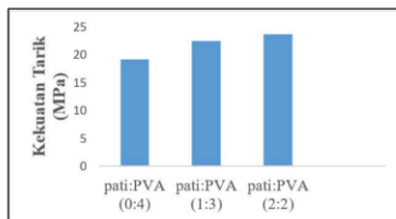
Gambar 2. Grafik Kekuatan Tarik Bioplastik Berdasarkan Rasio Pati : PVA Hasil pengukuran menunjukkan bahwa nilai kekuatan tarik masing-masing sampel berturut-turut adalah:
