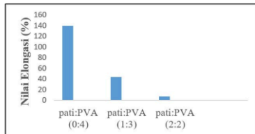
Gambar 3. Grafik Nilai Elongasi Bioplastik
