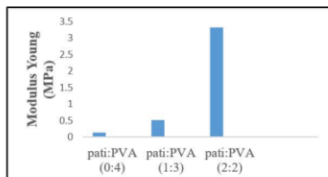
Gambar 4. Grafik Nilai Modulus Young Bioplastik
