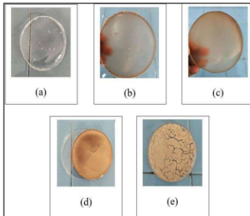
Gambar 1. Tampilan Bioplastik dari Campuran Pati : PVA
