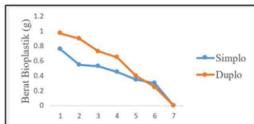
Gambar 5. Grafik Hasil Uji Biodegradasi Bioplastik
