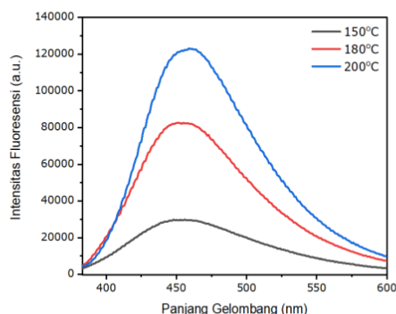
Gambar 3. Intensitas fluoresensi N-CDs pada berbagai variasi suhu
